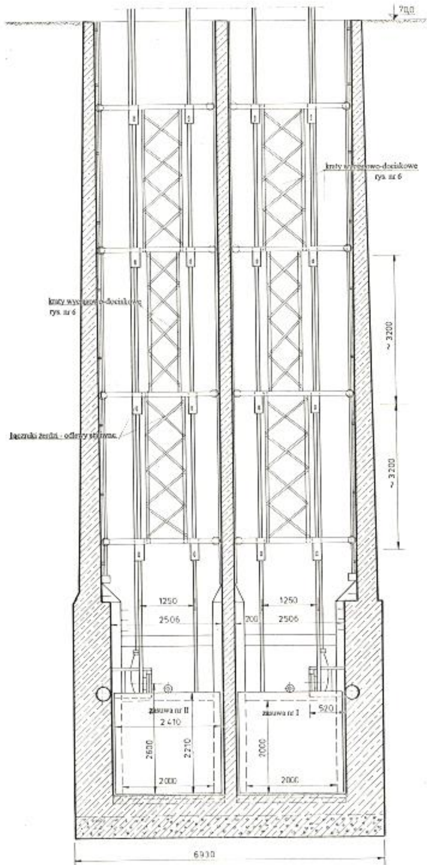
Rysunek 2. Przekrój pionowy z widokiem na zasuwy odwodne.
